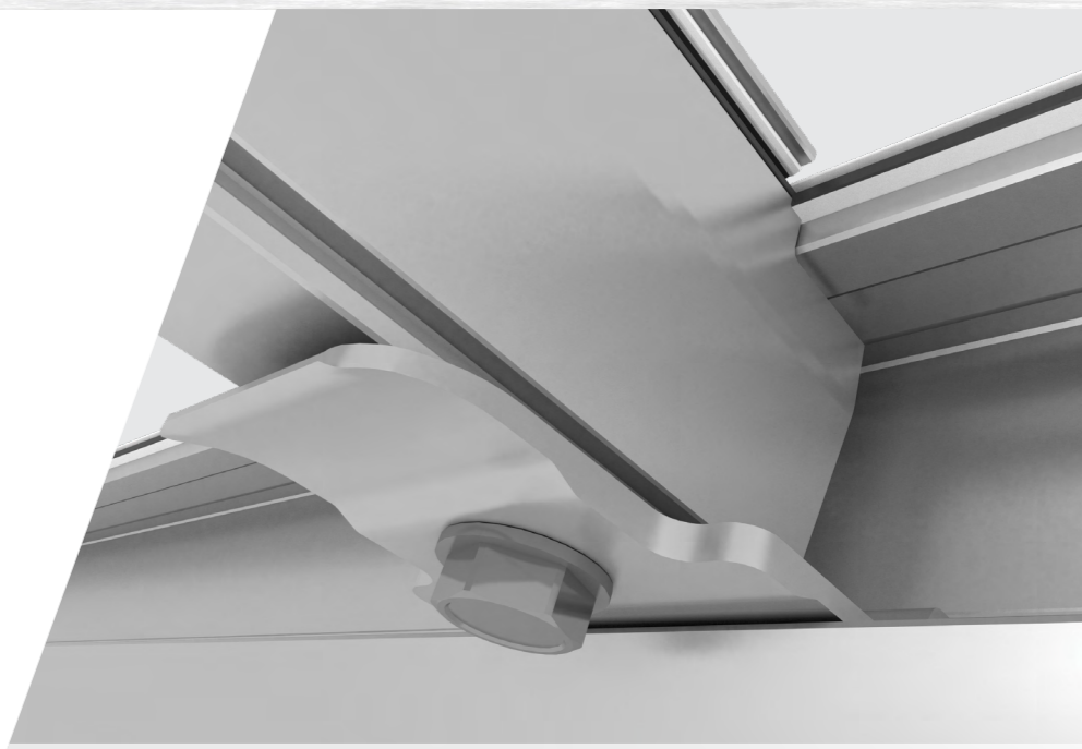
Dekroede wordt stormvast gemonteerd met behulp van de fixeerhaak. Nieuwe generatie VGS in de dekroede voor verbeterde afdichting.
